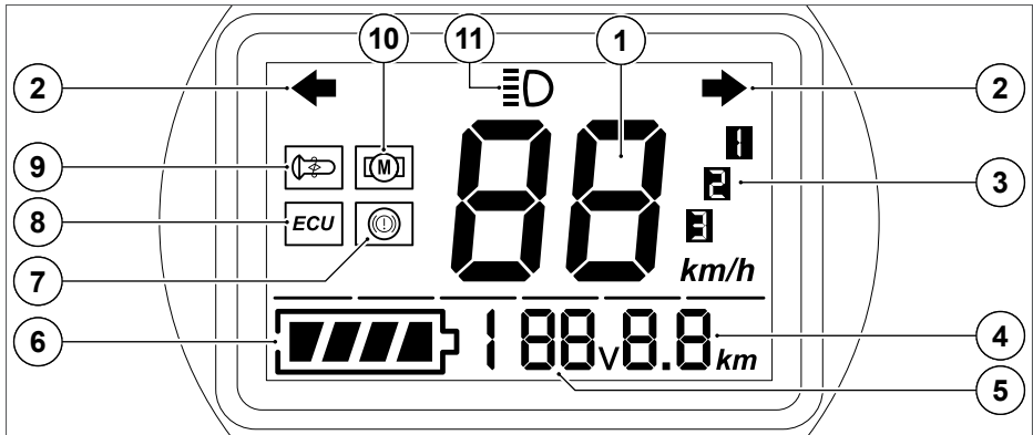
Abb. 4 Übersicht Instrumentenanzeige (Beispieldarstellung)
